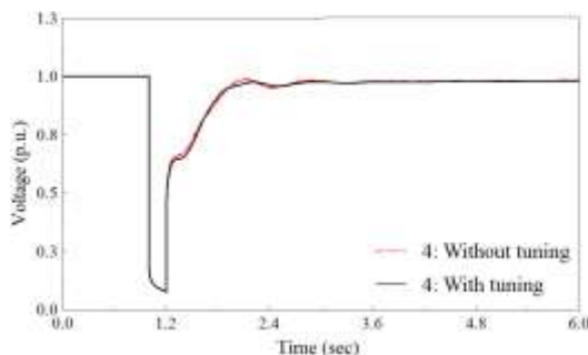
شکل (۱۷): ولتاژ باس ۴ (DG1) به‌ازای خطای F1
