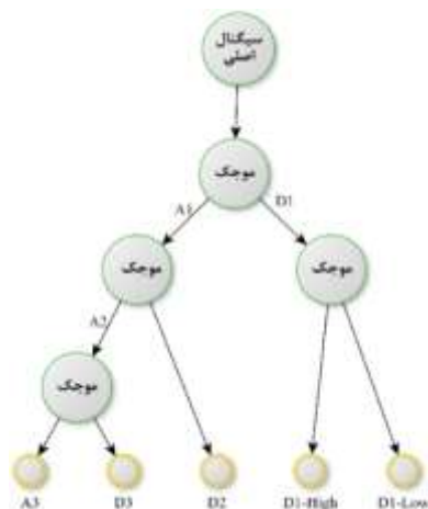
شکل (۱): مراحل شکستن سیگنال ورودیاز موجک چندمرحله‌ای
