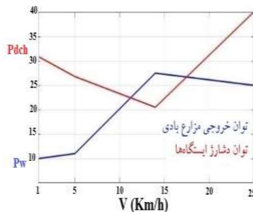
شکل (۸): مقایسه توان خروجی مزارع بادی و توان دشارژ ایستگاه‌ها
