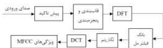
شکل (۴): بلوک دیاگرام محاسبه MFCC
