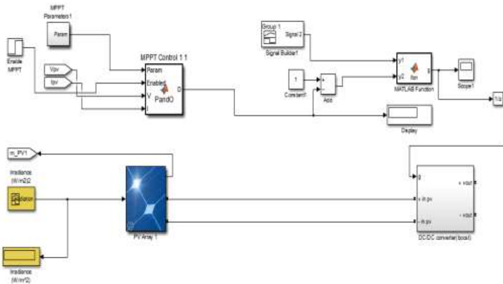
شکل (۴): سیستم تعقیب کننده ماکزیم توان سلول خورشیدی
