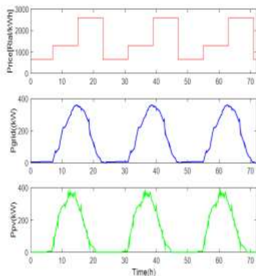
شکل (۱۴): نمودار هزینه، توان خروجی شبکه، توان تولیدی سلول خورشیدی مربوط به سناریوی ششم
