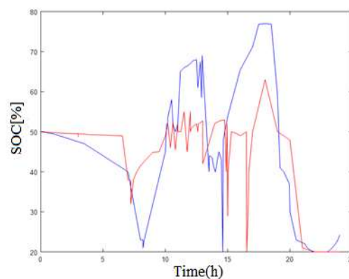
شکل (۱۵): نمودار درصد شارژ باتری‌ها با کنترل‌کننده پیشنهادی (نمودار قرمز مربوط به باتری کوچک و نمودار آبی مربوط به باتری بزرگ است).
