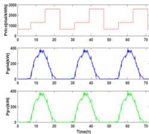
شکل (۸): نمودار هزینه، توان خروجی شبکه، توان تولیدی
