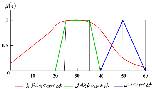
شکل (۱): توابع عضویت.
