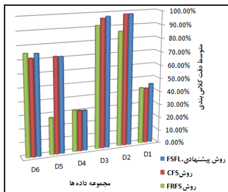
شکل (۶): نمودار مقایسه ای روش FSFL با روش های دیگر.
