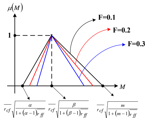
شکل (۴): نمایشی از \mu(M) با استفاده از F.
