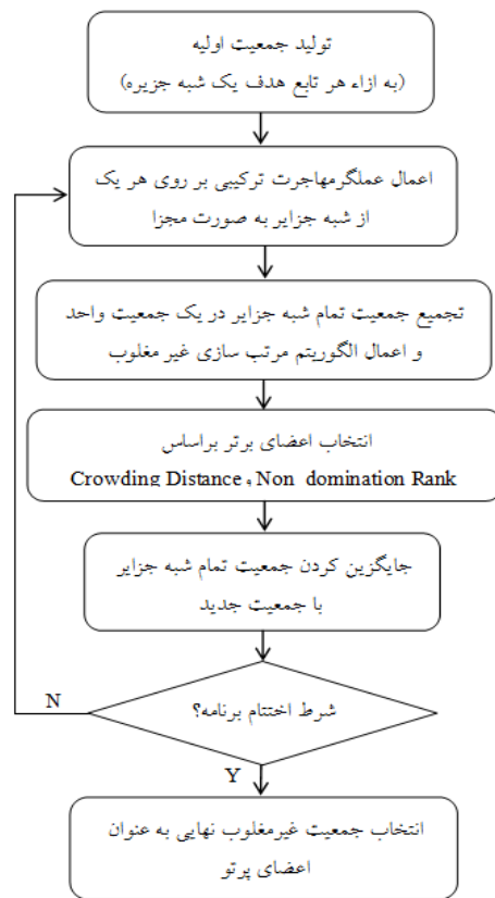
شکل ۲: فلوجارت الگوریتم پیشنهادی
