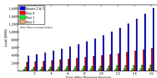
شکل (۵): منحنی بار شین‌های شکل (۴) در سال‌های پس از افق طراحی
