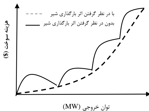
شکل (۵): منحنی ورودی-خروجی تحت تأثیر بارگذاری شیر [۱۳]
