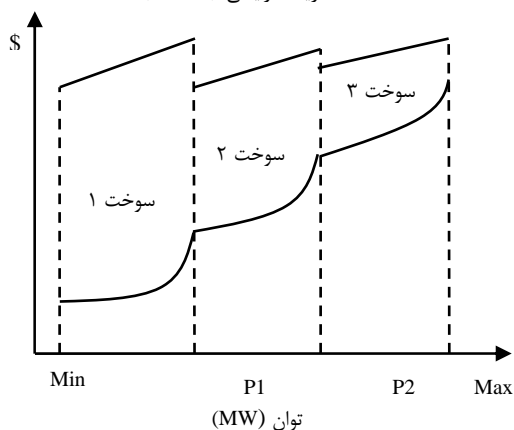
شکل (۶): تابع هزینه سوخت از واحد تولید حرارتی که چندین سوخت متفاوت استفاده می‌کند [۱۳]
