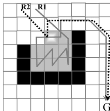
شکل (۱۰): اعمال قاعده بهبود یافته اتوماتا به یک سیستم دو رباتی. R1 ناحیه تعمر را قبل از رسیدن R2 ترک کرده است.
